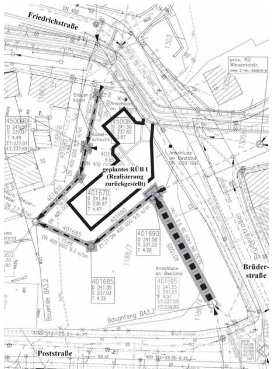
„Provisorischer Zusammenschluss des Hauptsammlers (gestrichelte Darstellung)“
